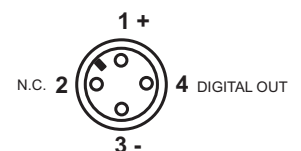
Uscita digitale Digital output
